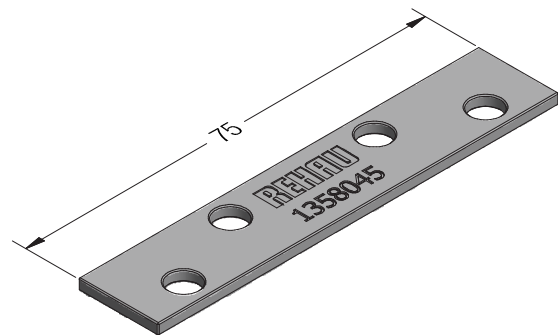
Montageplatte Pfosten 96 und 124 SYNEGO®
